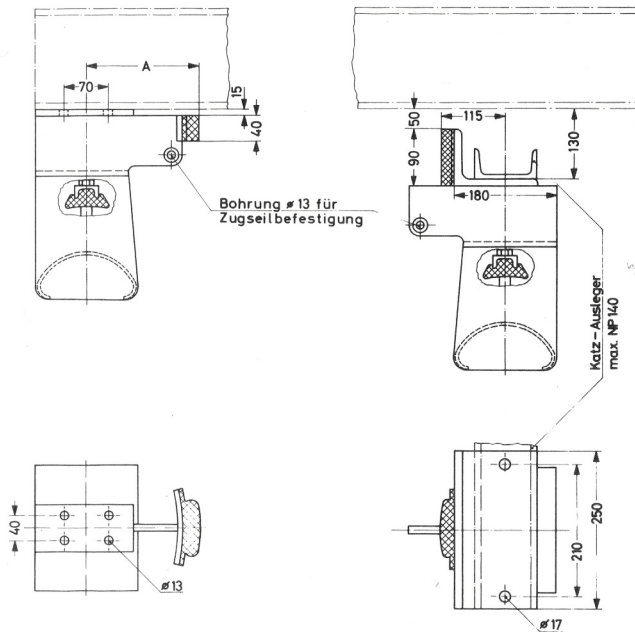
Endklemme für die Laufschiene EL
